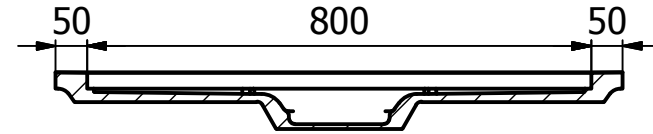
B-B ( 1/12 )
