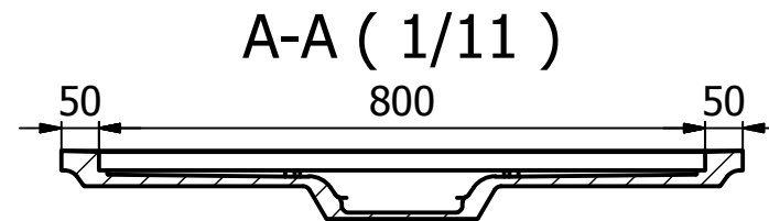
A-A ( 1/11 )
