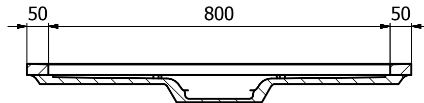
A-A ( 1/9 )
