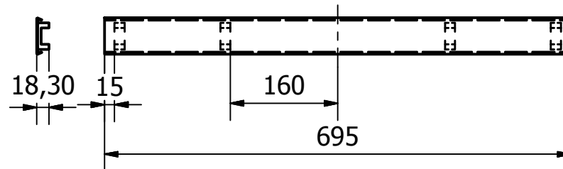
Doucherooster 695mm GC gespoten
