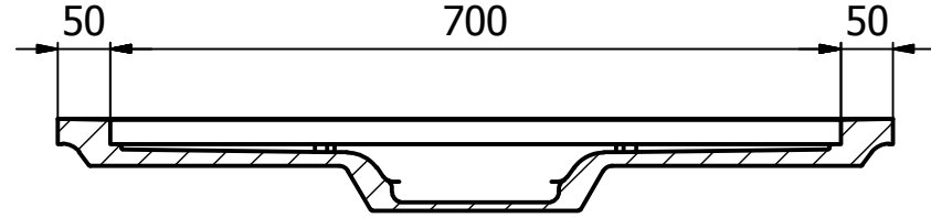
A-A ( 1/8 )
